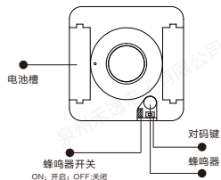
(图2: 底盒示意图)
